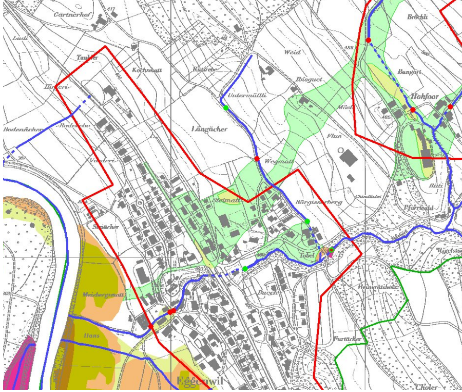
Fliesstiefen HQ300 nach Massnahmen
