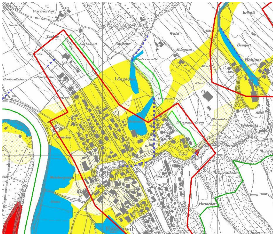
Gefahrenkarte vor Massnahmen
