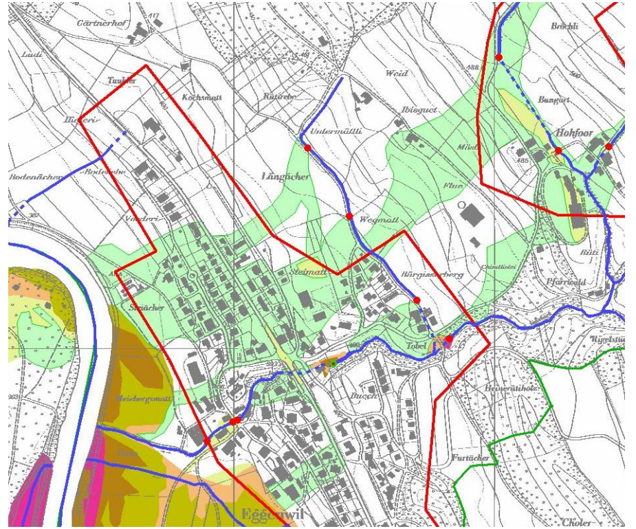
Fliesstiefen EHQ nach Massnahmen
