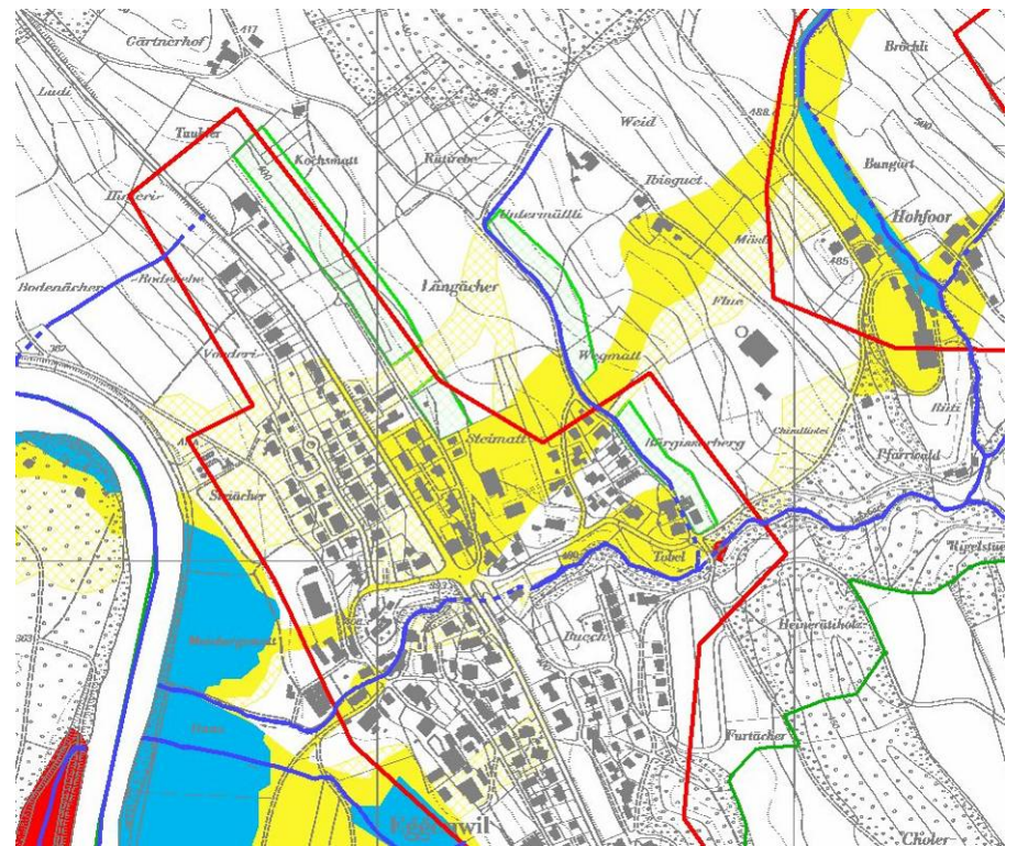
Gefahrenkarte nach Massnahmen
