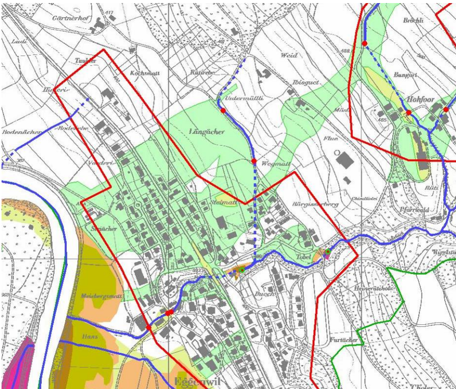
Fliesstiefen HQ300 vor Massnahmen
