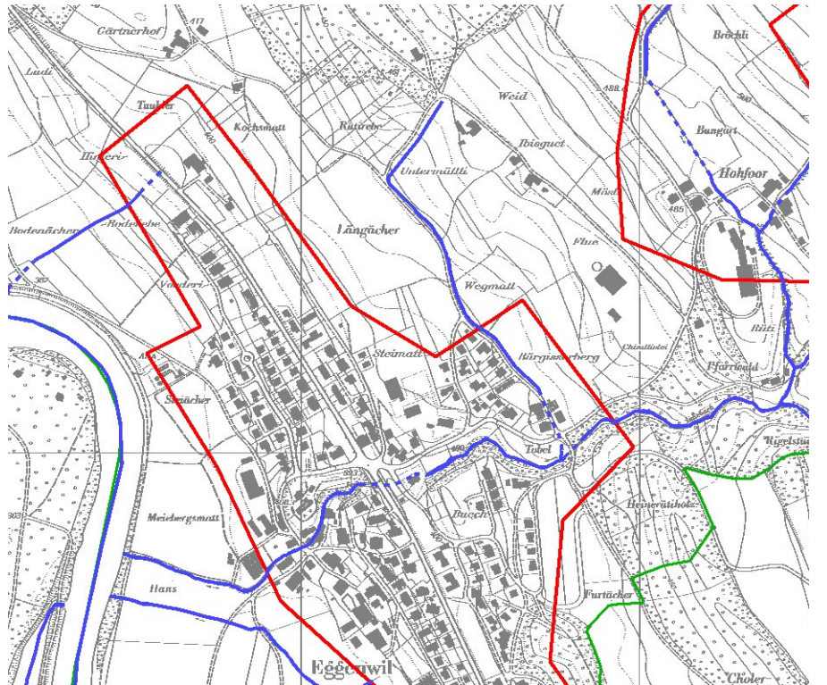
Schutzdefizite nach Massnahmen
