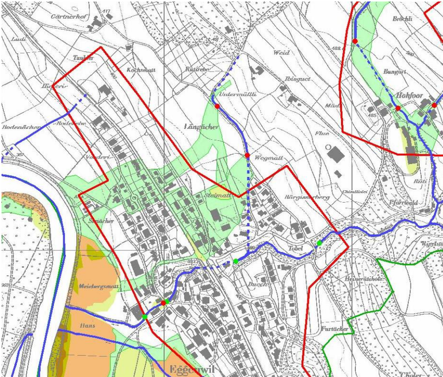
Fliesstiefen HQ100 vor Massnahmen
