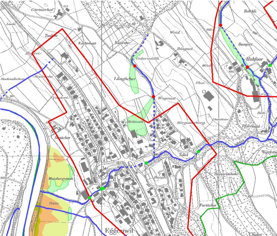
Fliesstiefen HQ30 vor Massnahmen
