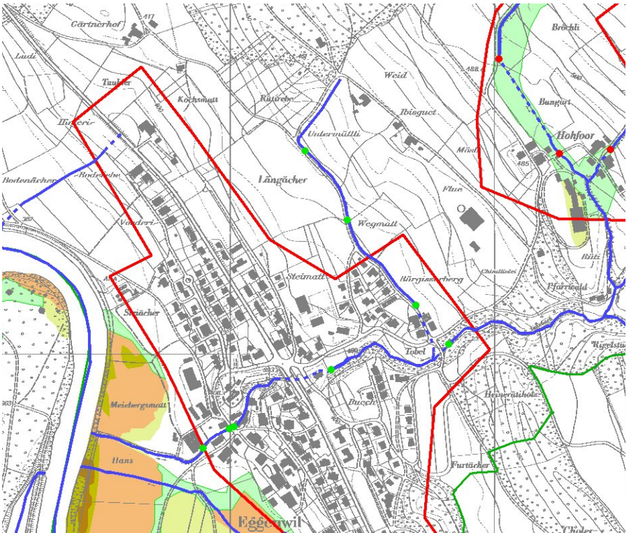
Fliesstiefen HQ100 nach Massnahmen
