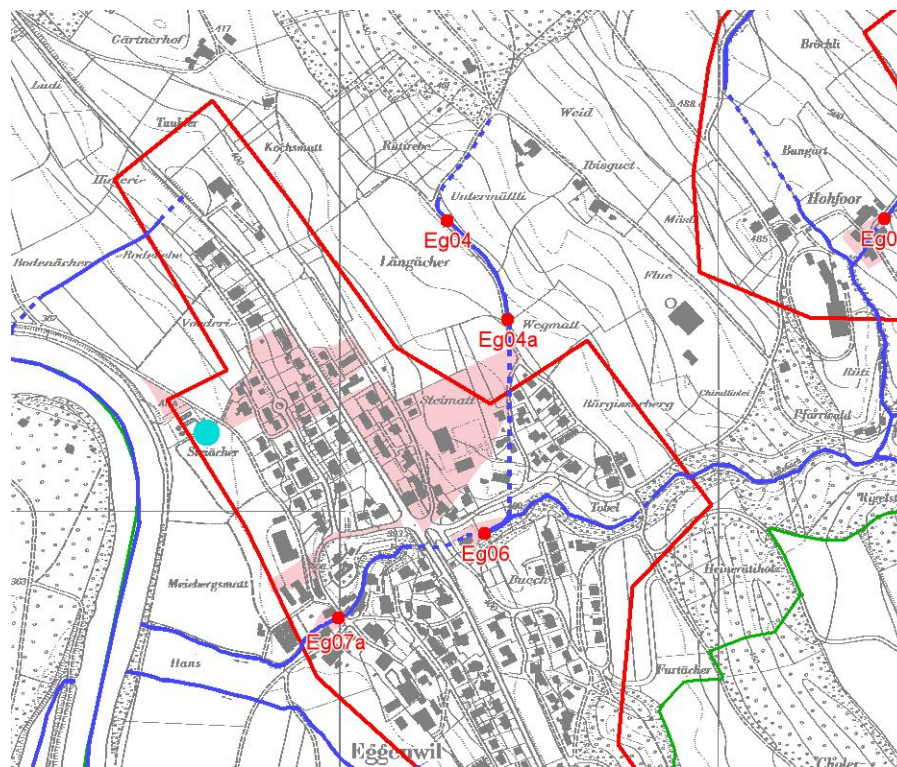
Schutzdefizite vor Massnahmen
