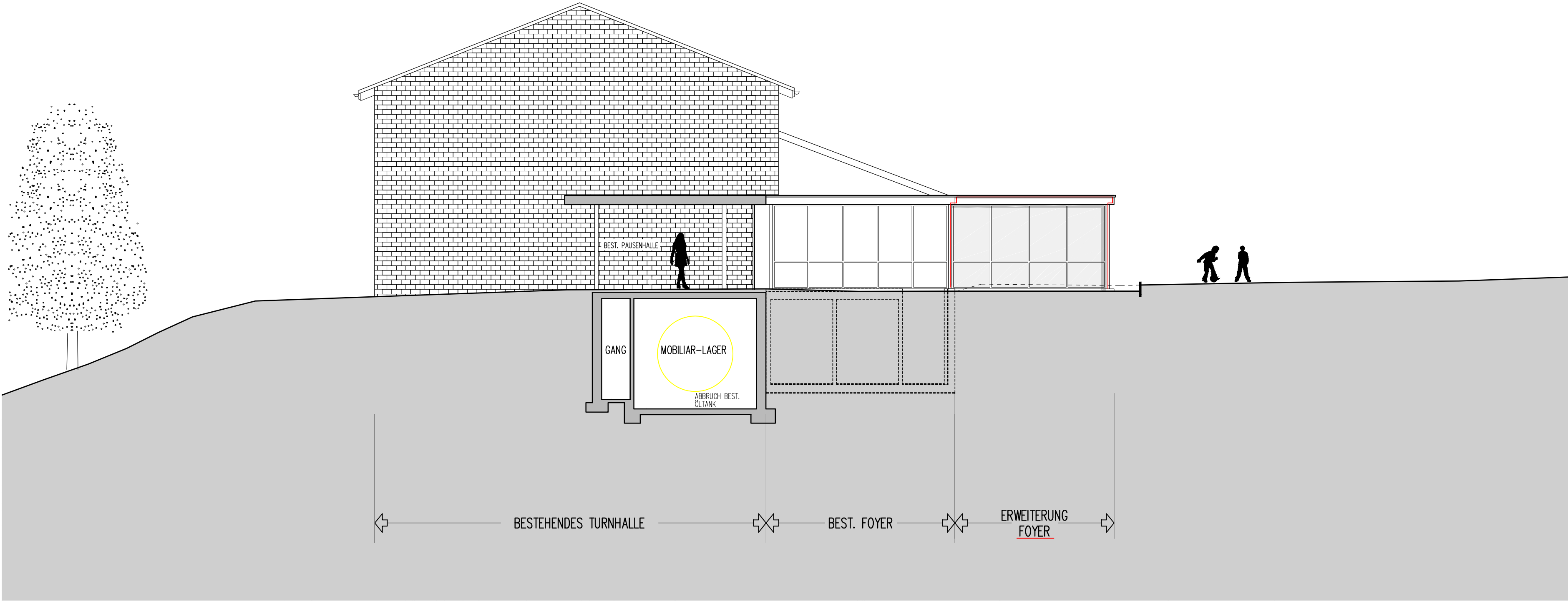
SÜDANSICHT
