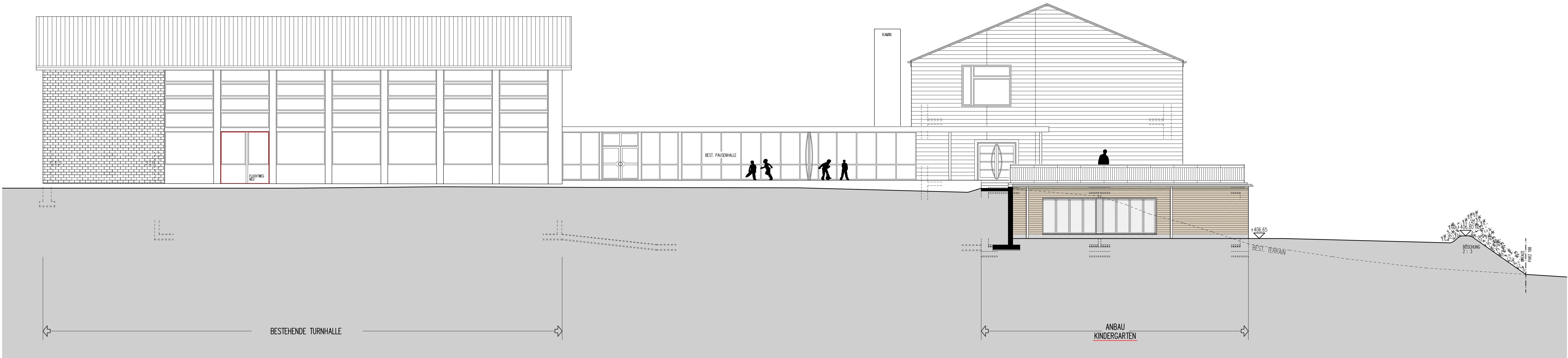
WESTFASADE
